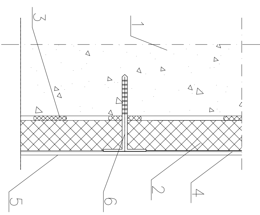
Szczegół mocowania płyt styropianowych
